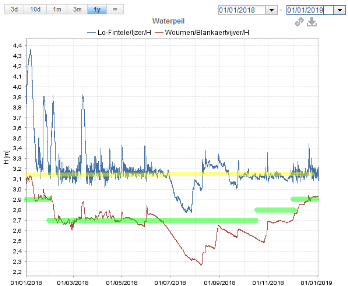
Figuur 2: Waterpeil IJzer en Blankaertvijver 2018
