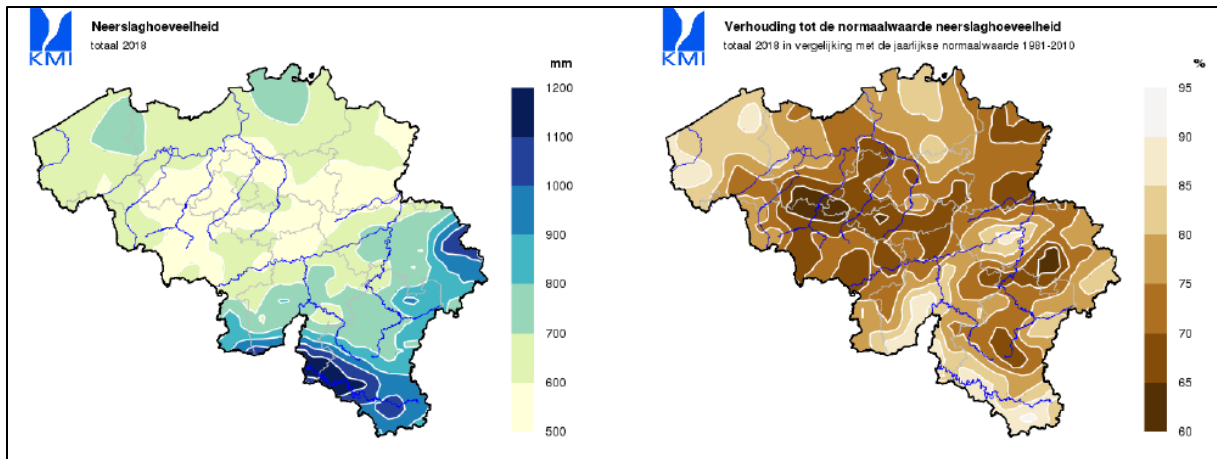
Figuur 3: Totale neerslaghoeveelheid en afwijking totale neerslag t.o.v. normale neerslag
