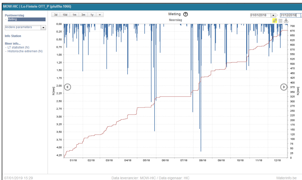
Figuur 1: Cumulatieve neerslagverdeling 2018
