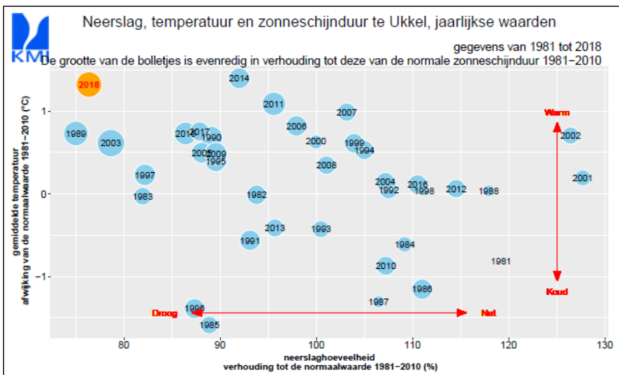
Figuur 4: Gemiddelde temperatuur vs. neerslaghoeveelheid
