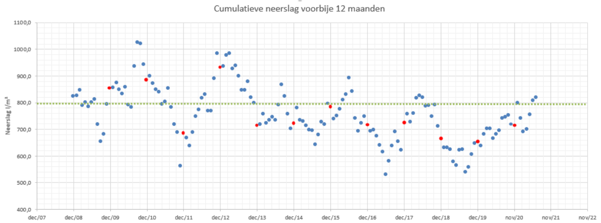
Figuur 4: Cumulatieve 12-maandelijke neerslag
