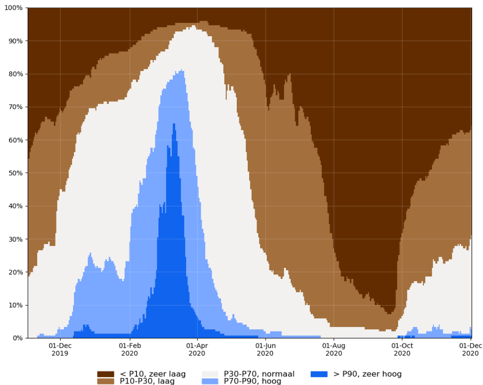
Figuur 4: Freatisch grondwaterstandindicator Vlaanderen
