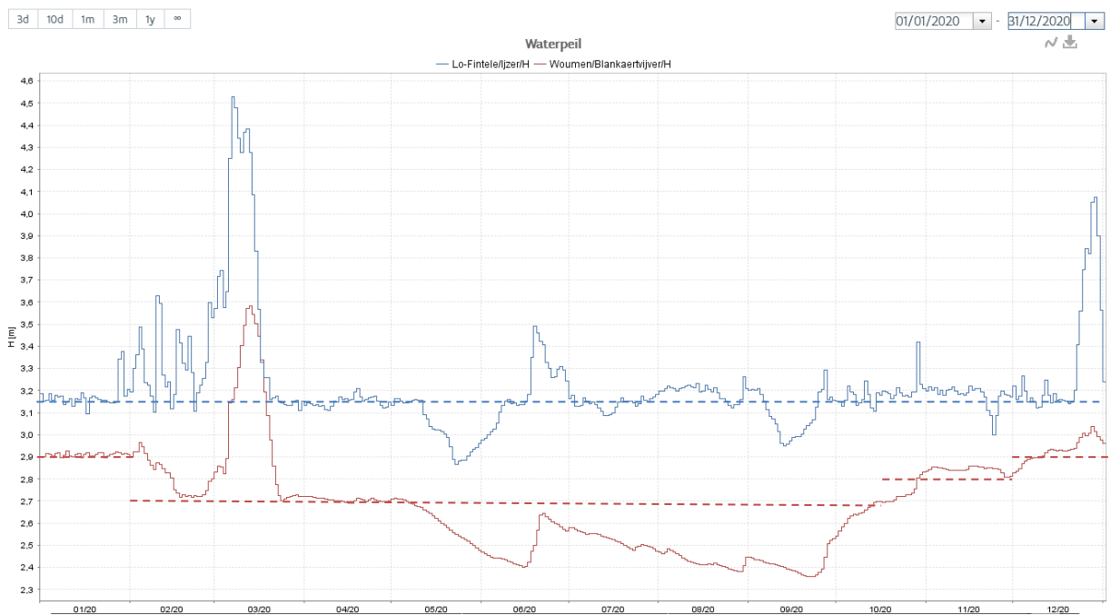
Figuur 5: Waterpeil IJzer en Blankaartvijver 2020
